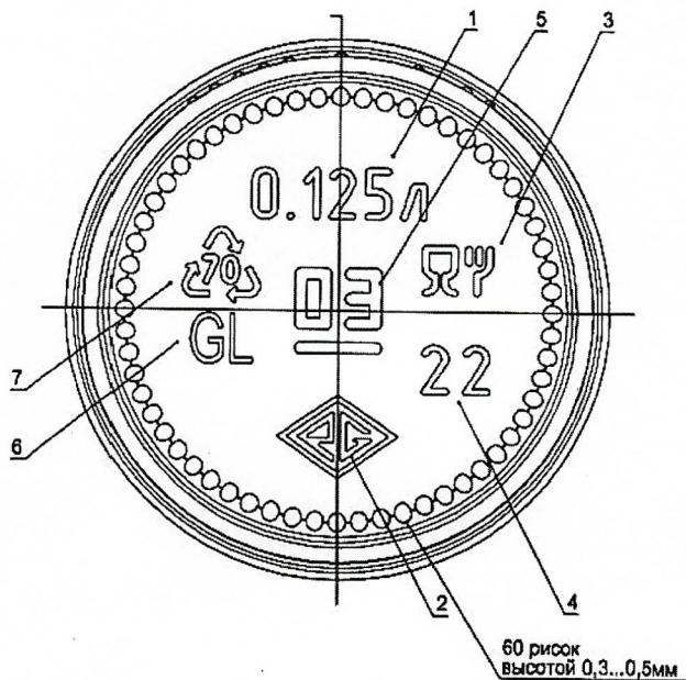
ВИД СНИЗУ
