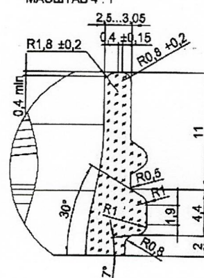
МЕСТНЫЙ В МАСШТАБ 4:1
