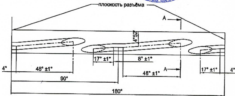
Развертка формирующей поверхности (фреза Ø 16)
