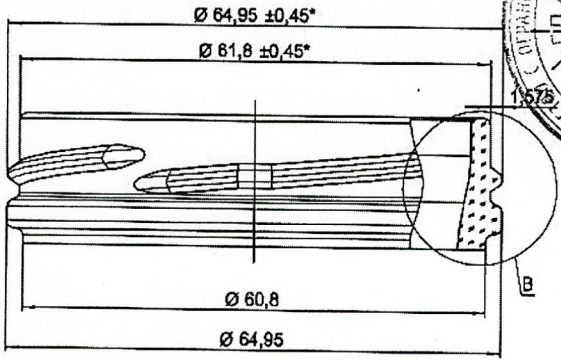
ВИД СПЕРЕДИ
